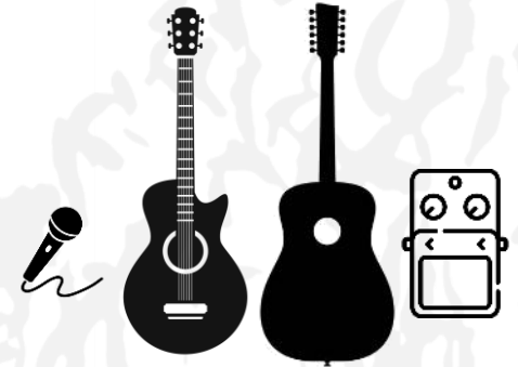
Andi Mikrofon an XR 18 (Ch 4) Gitarren 2x Klinke an Effektgerät Strom für Effektgerät Effektgerät Klinke an XR 18 (Ch 2)
